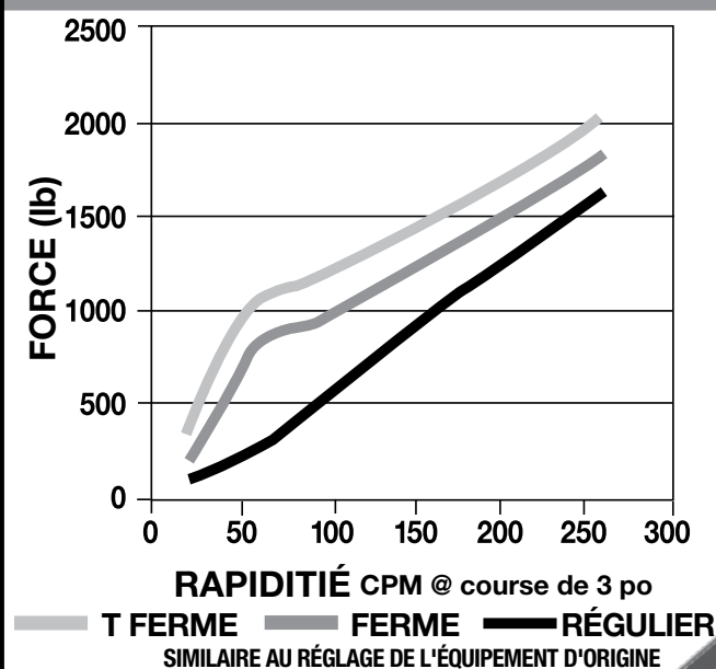
Force de détente des amortisseurs à gaz typiques comparée à celle de l'équipement d'origine
