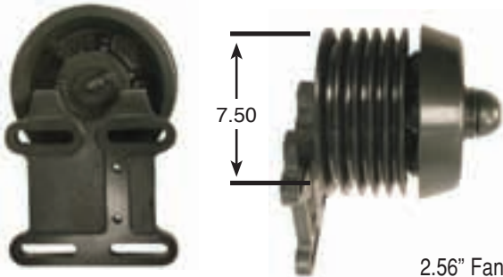
2.56" Fan Pilot
