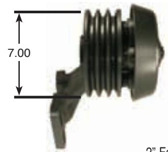
2" Fan Pilot
