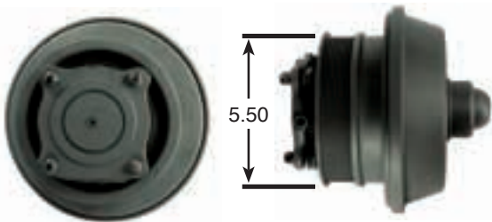
2.56" Fan Pilot
