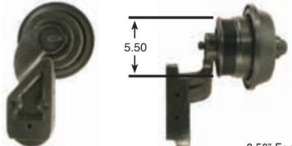
2.56" Fan Pilot
