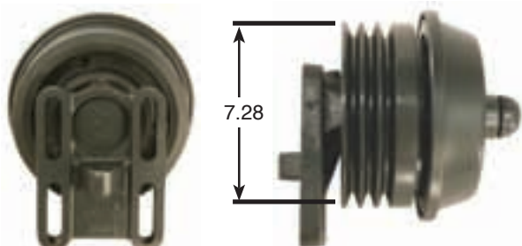
2.56" Fan Pilot
