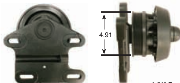
2.56" Fan Pilot
