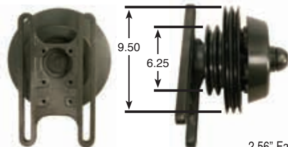
2.56" Fan Pilot
