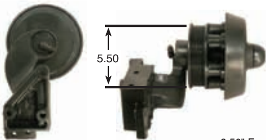
2.56" Fan Pilot
