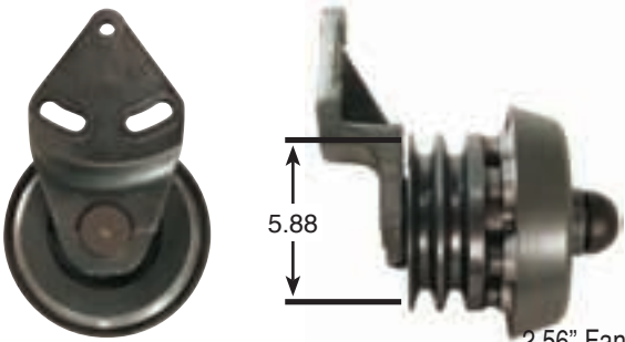
2.56" Fan Pilot
