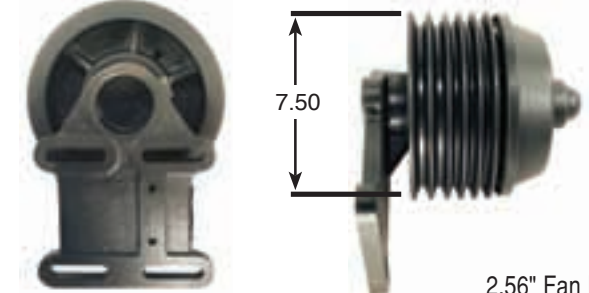
2.56" Fan Pilot
